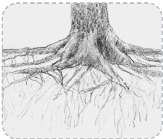
Flachwurzel – Fichte
